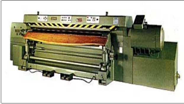
Hide Shaving Machine Tıraşlama makinası
