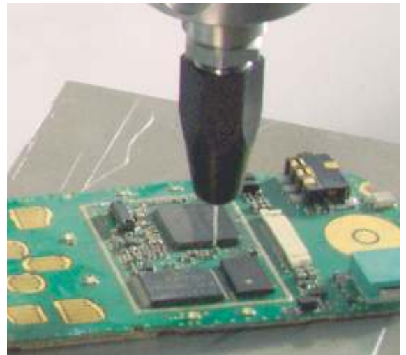
TS5440 - glob top. ►
